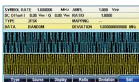
FSK
